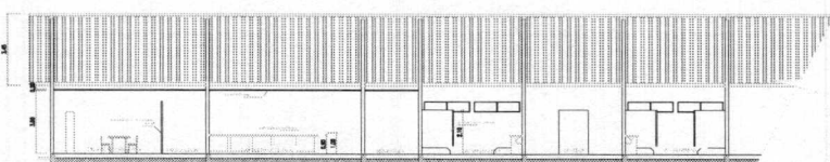
CORTE AA' ESCALA... 1/125
