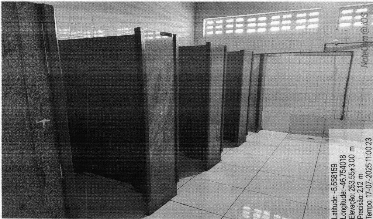
IMAGEM 11: Troca do revestimento cerâmico, manutenção das divisórias em granito e substituição das paredes de cobogó por janelas de vidro.
