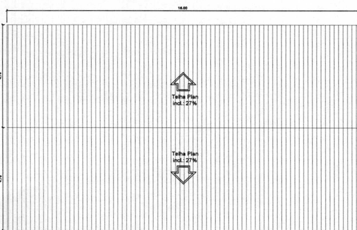
02 PLANTA DE COBERTURA C/ AMPLIAÇÃO ESCALA = 1:100
