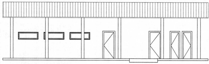
02 FACHADA C/ AMPLIAÇÃO ESCALA = 1/100
