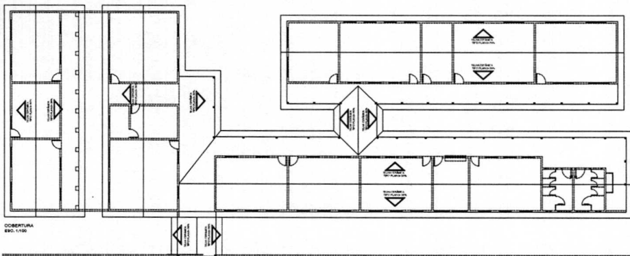
PLANTA DE COBERTURA ESQ. 1:100
