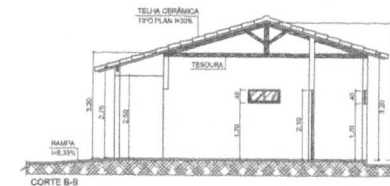
CORTE B-B ESC. 1/50
