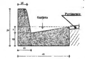
2 Detalhe Corte Sarjeta 1:10
