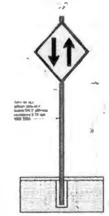
DETALHE - PLACA A-25 ADVERTENCIA DUPLA SENTIDO DE CIRCULAÇÃO
